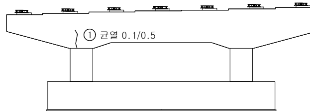
우측면
